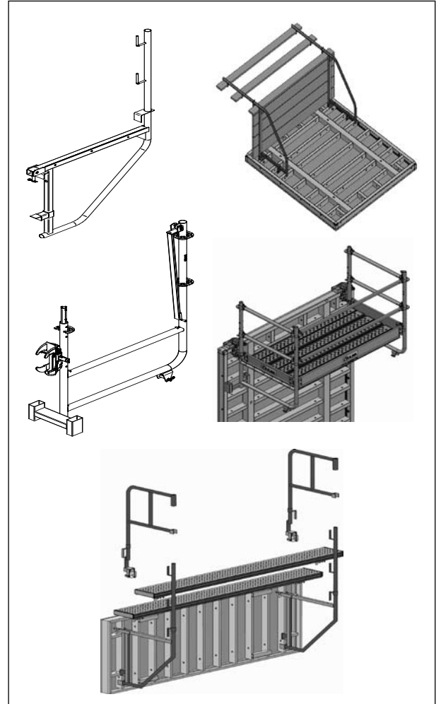
Figura 8. Tipos de ménsulas/consolas de trabajo
